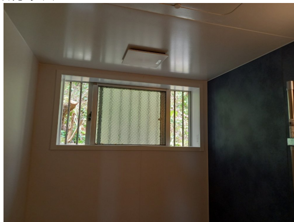
6.ガラス
