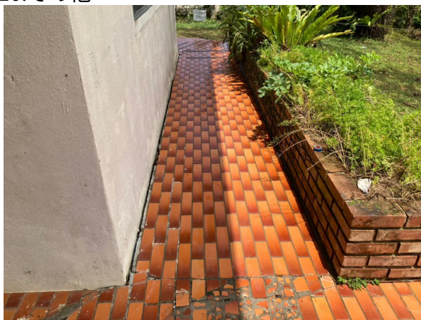
10.その他
